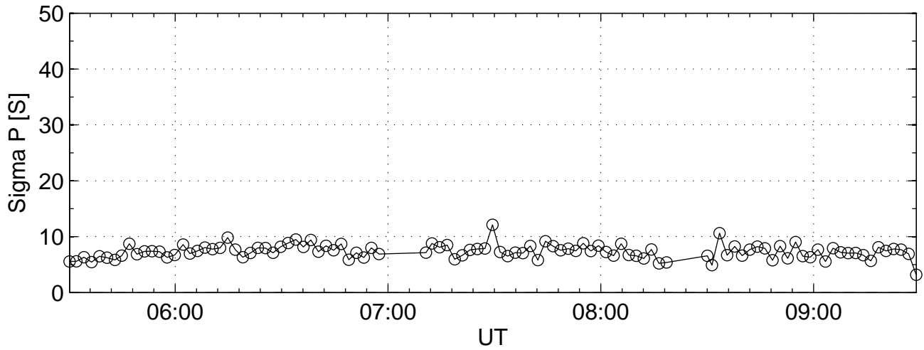
2002-07-16 tau0@42m Sigma P
