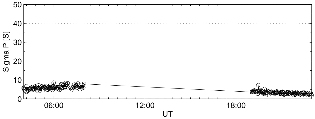
2002-07-31 tau0@42m Sigma P
