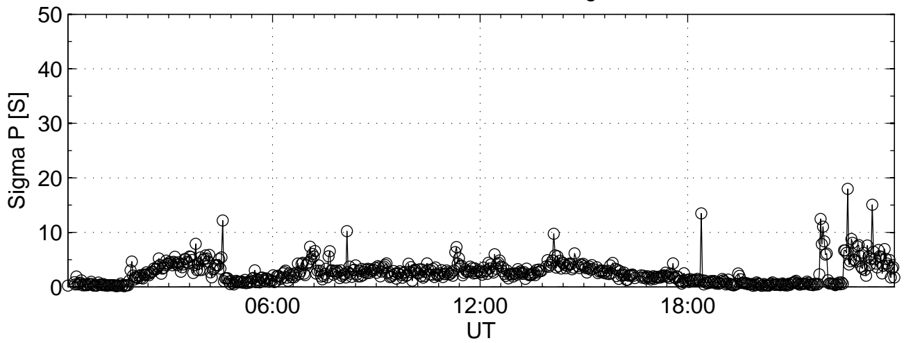
2003-03-21 tau0@42m Sigma P
