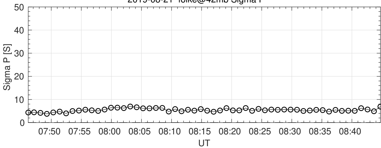
2019-08-21 folke@42mb Sigma P
