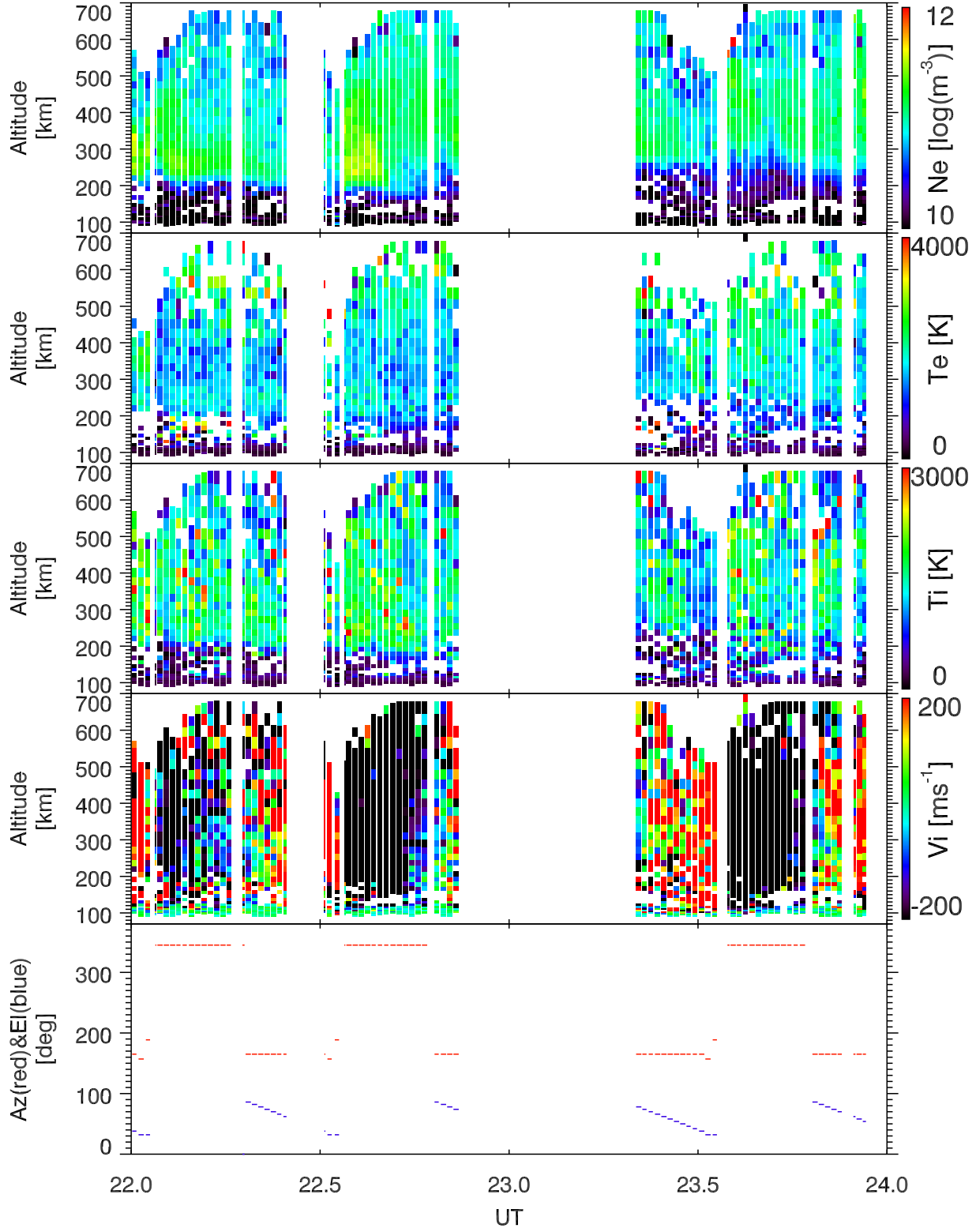
EISCAT 1998-10-20_22_24UT_gup3c_ant@32m.
