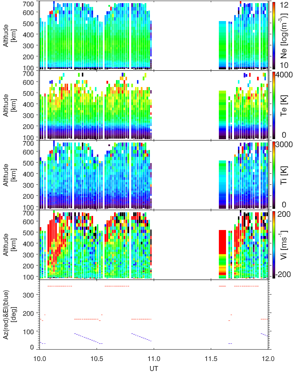
EISCAT 1999-04-22_10_12UT_gup3c_ant@32m.
