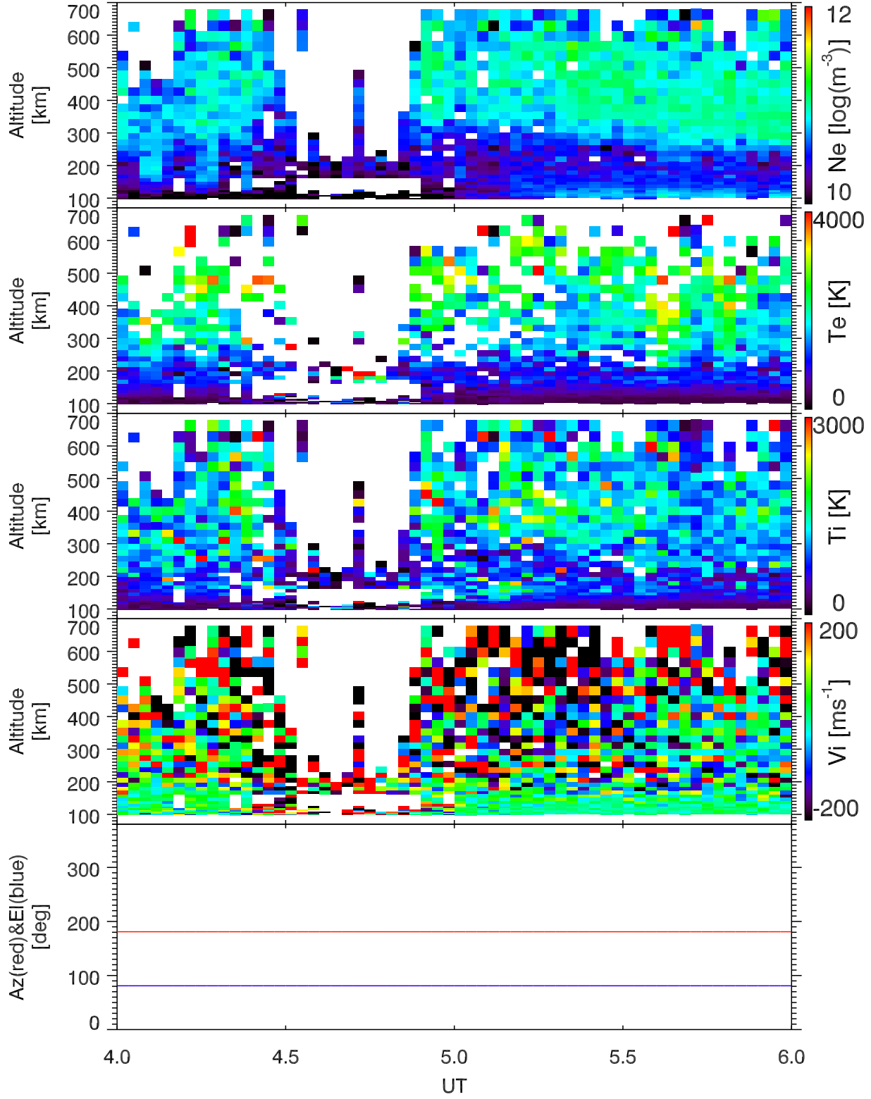
EISCAT 2000-02-08_04_06UT_gup3c_120@42m.
