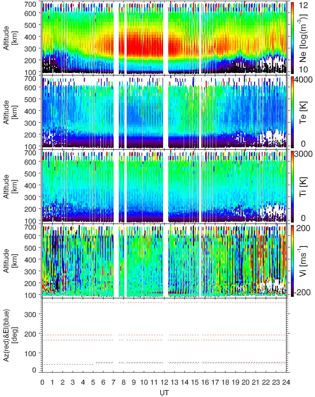
EISCAT 2000-03-16_00_24UT_gup3c_ant@32m.
