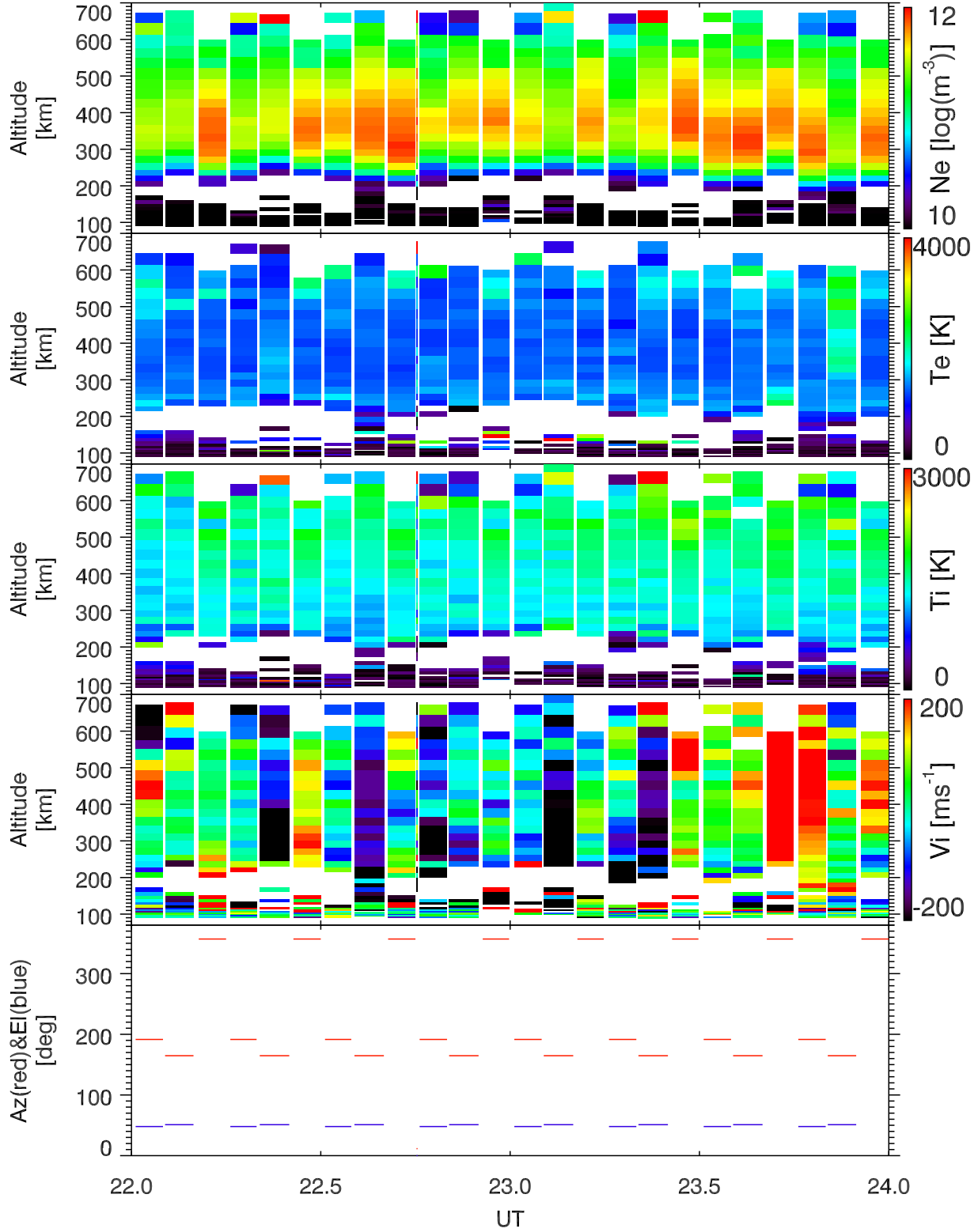
EISCAT 2000-03-16_22_24UT_gup3c_ant@32m.
