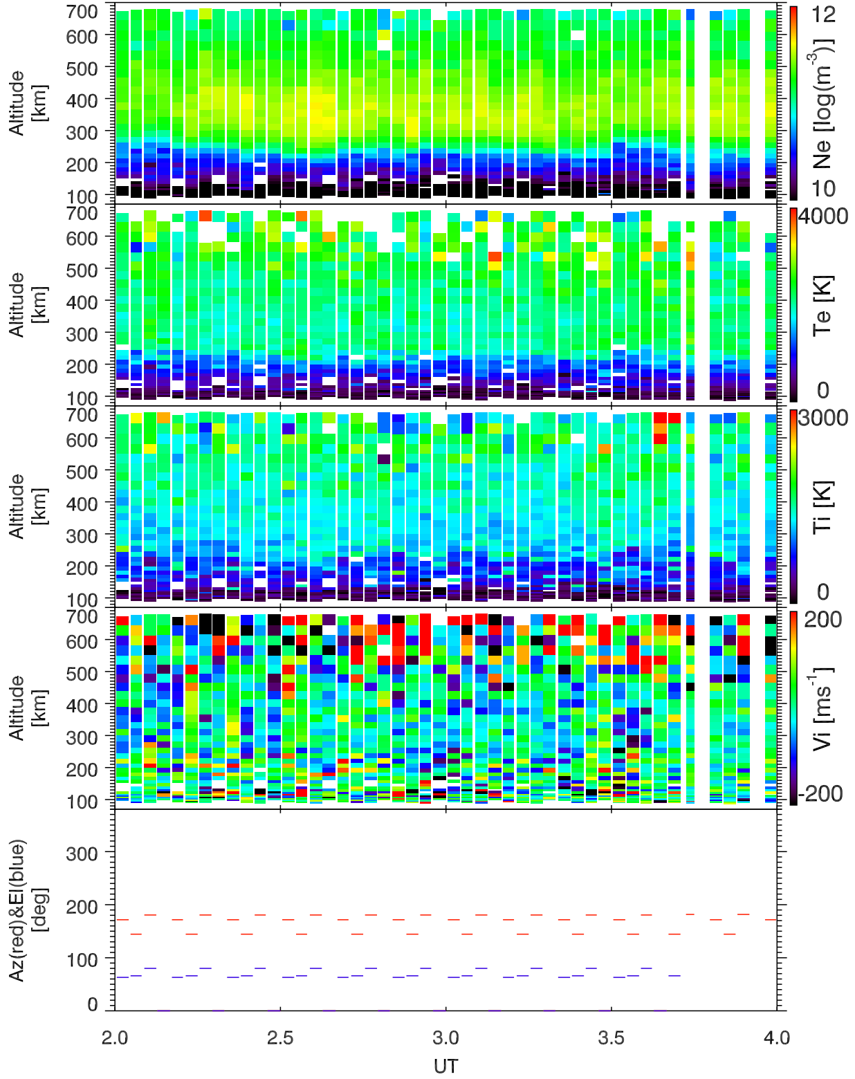
EISCAT 2000-03-18_02_04UT_gup3c_ant@32m.
