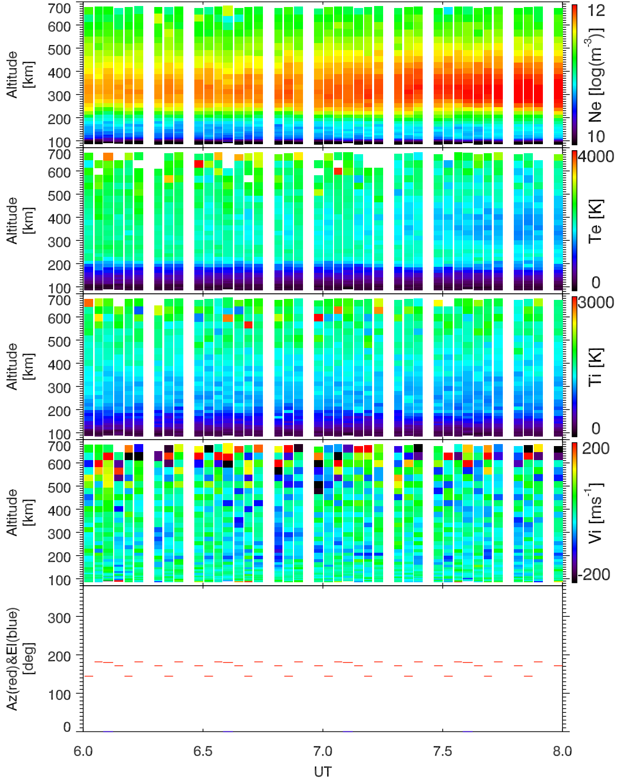
EISCAT 2000-03-18_06_08UT_gup3c_ant@32m.
