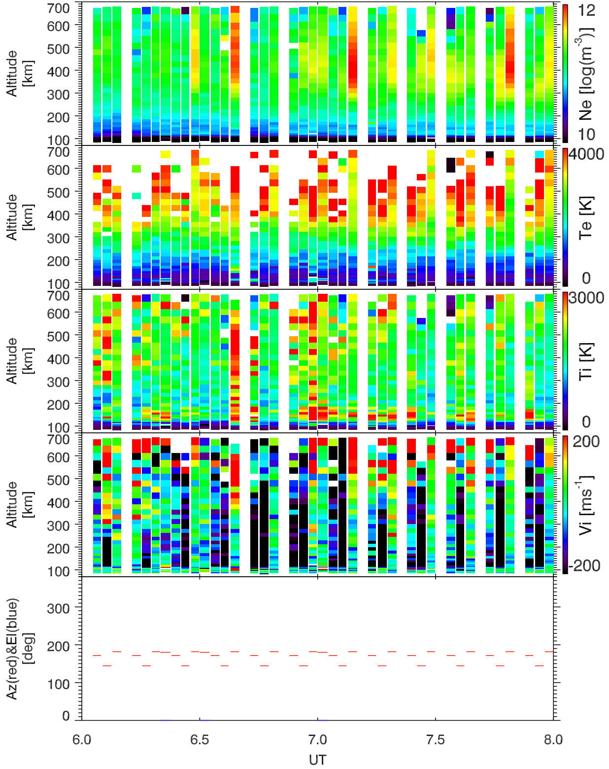
EISCAT 2000-03-19_06_08UT_gup3c_ant@32m.
