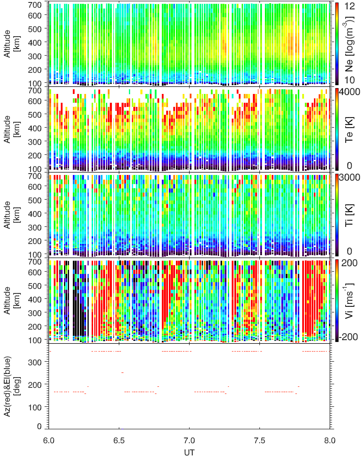
EISCAT 2000-04-12_06_08UT_tau0_ant@32m.
