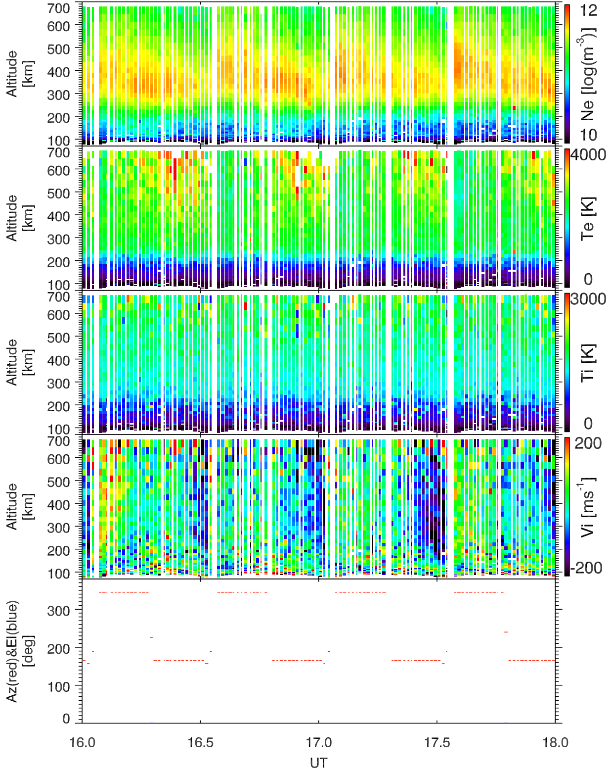
EISCAT 2000-04-12_16_18UT_tau0_ant@32m.
