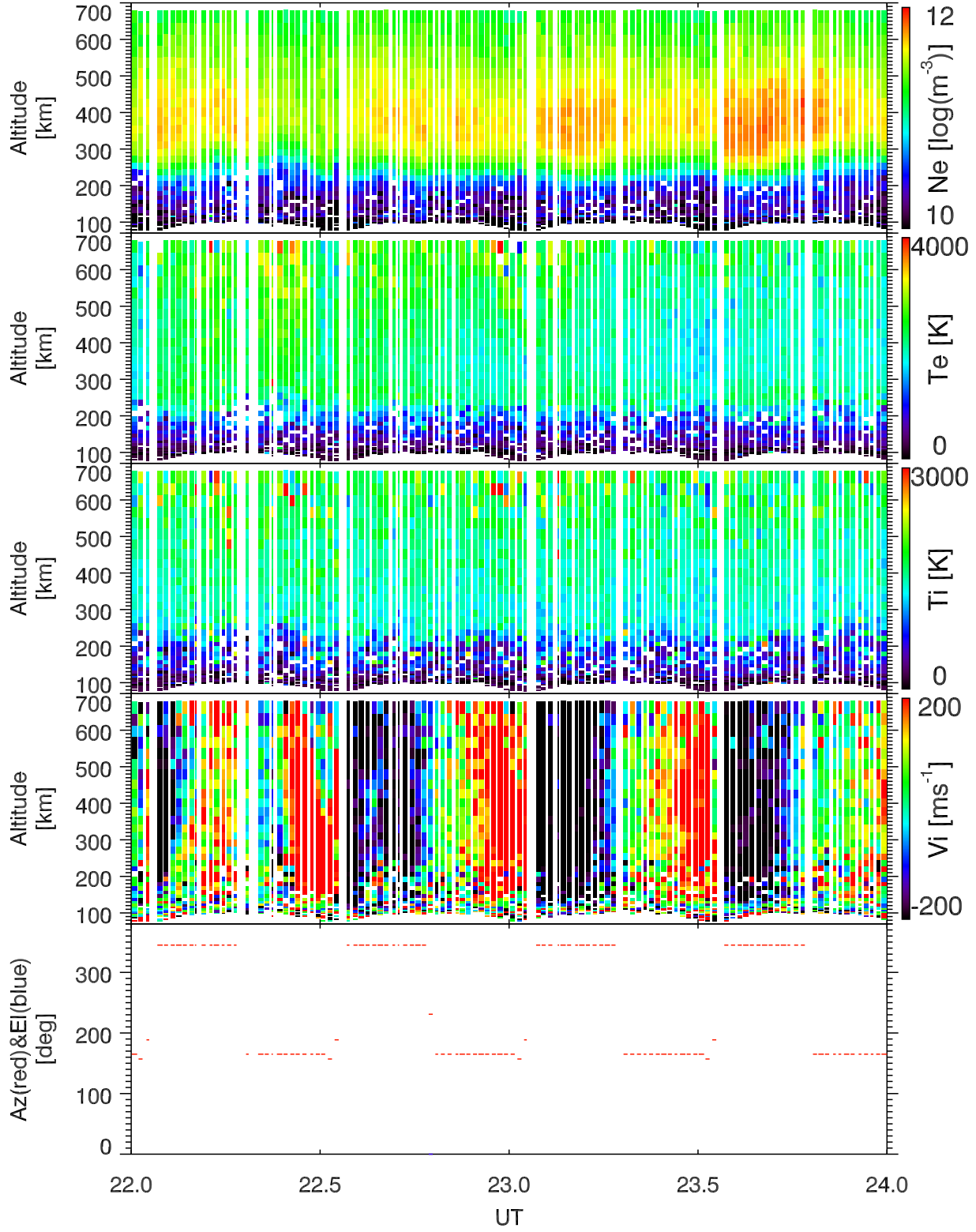
EISCAT 2000-04-12_22_24UT_tau0_ant@32m.
