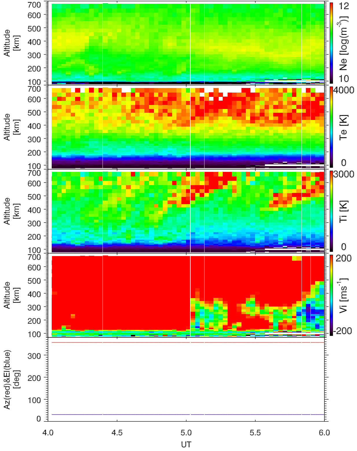
EISCAT 2000-07-19_04_06UT_tau0_120@32m.
