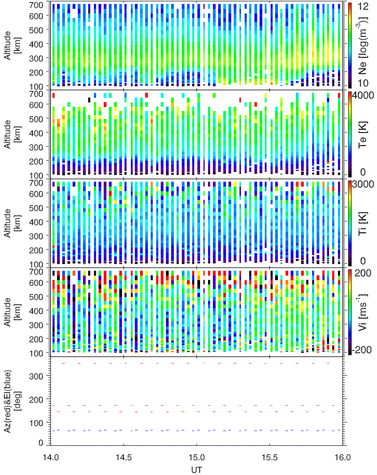
EISCAT 2001-02-17_14_16UT_tau0_ant@32m.
