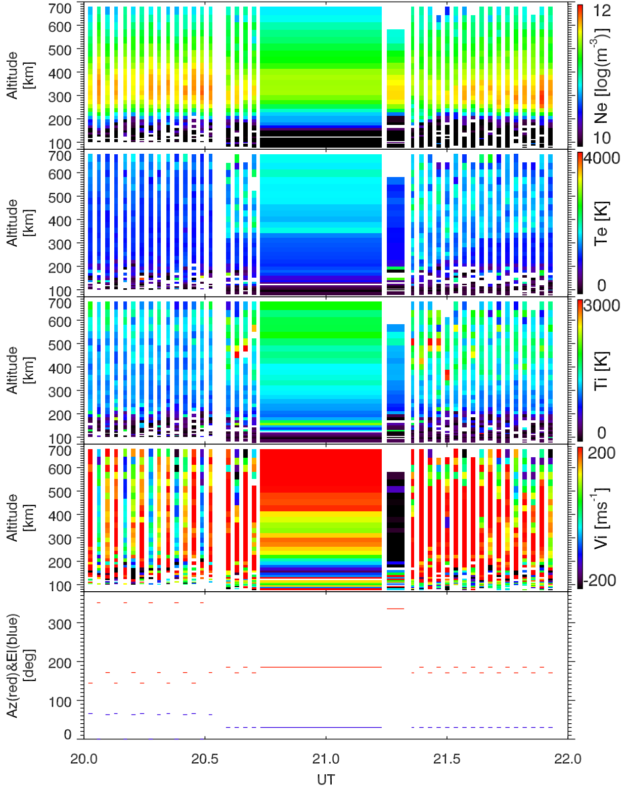
EISCAT 2001-02-17_20_22UT_tau0_ant@32m.
