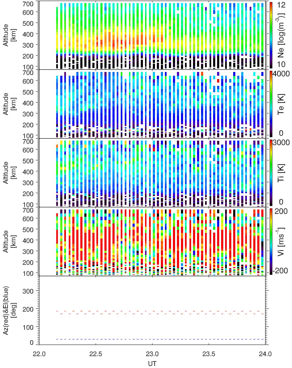
EISCAT 2001-02-17_22_24UT_tau0_ant@32m.
