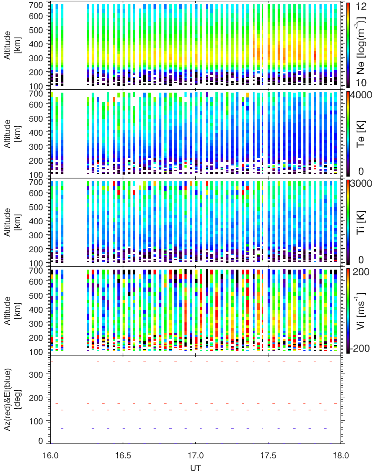
EISCAT 2001-02-18_16_18UT_tau0_ant@32m.
