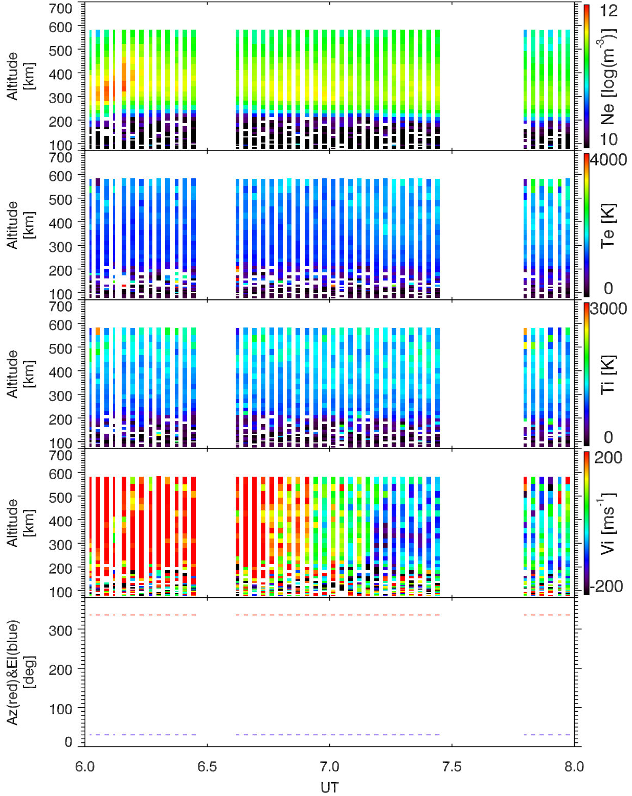
EISCAT 2001-02-19_06_08UT_tau0_ant@32m.
