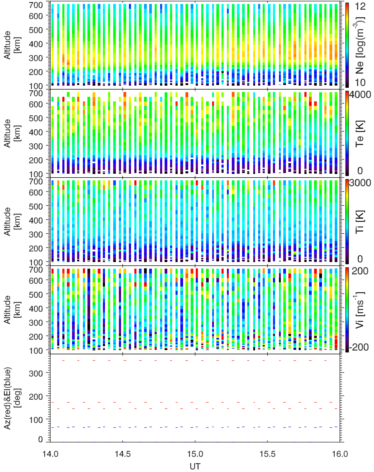
EISCAT 2001-02-20_14_16UT_tau0_ant@32m.
