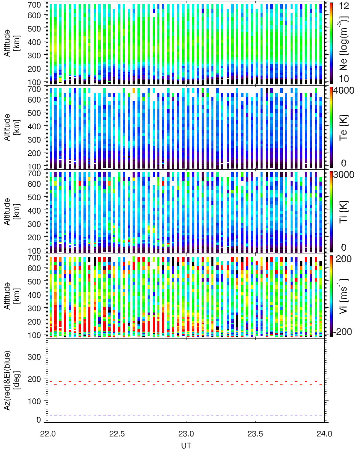
EISCAT 2001-02-21_22_24UT_tau0_ant@32m.
