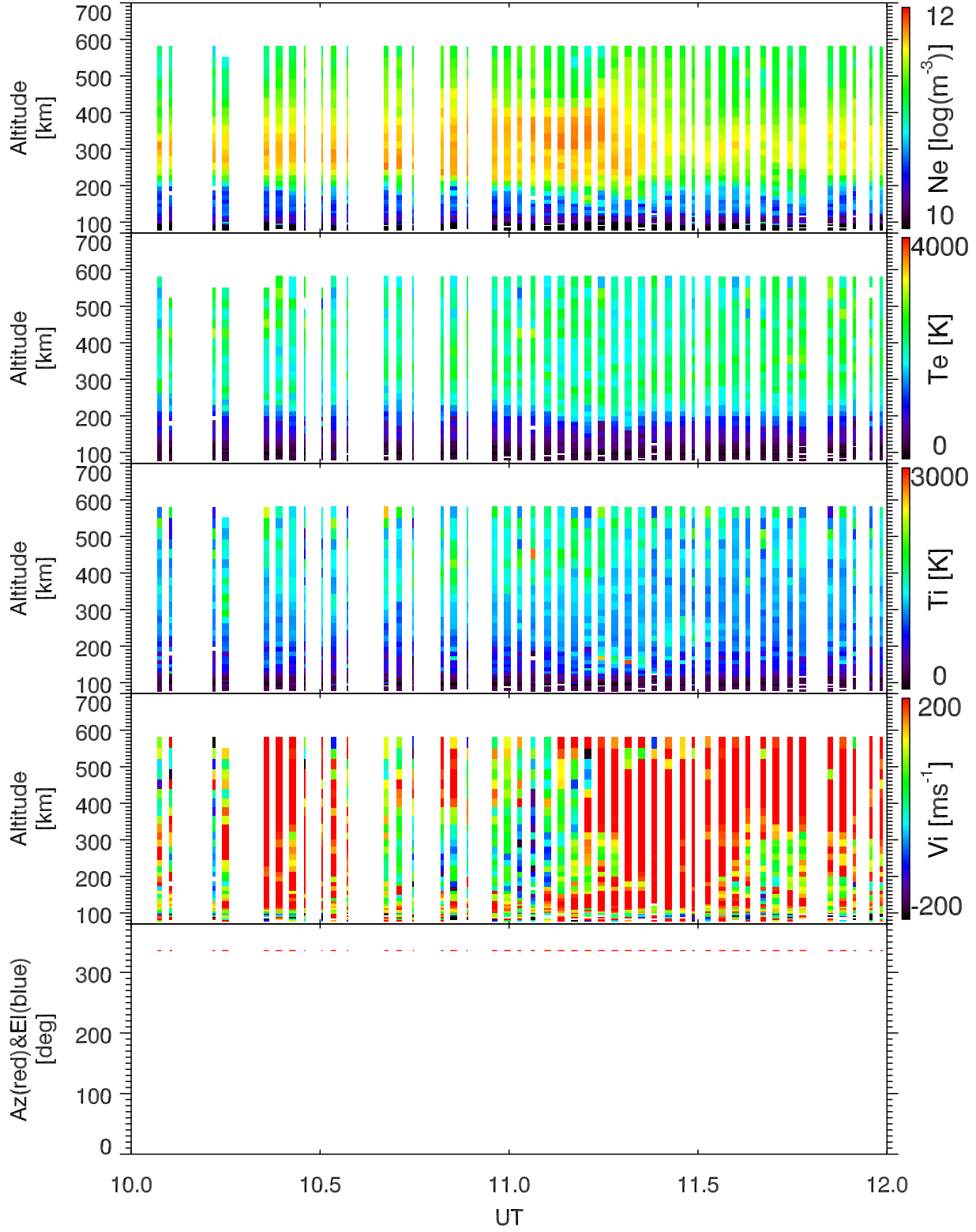
EISCAT 2001-02-22_10_12UT_tau0_ant@32m.
