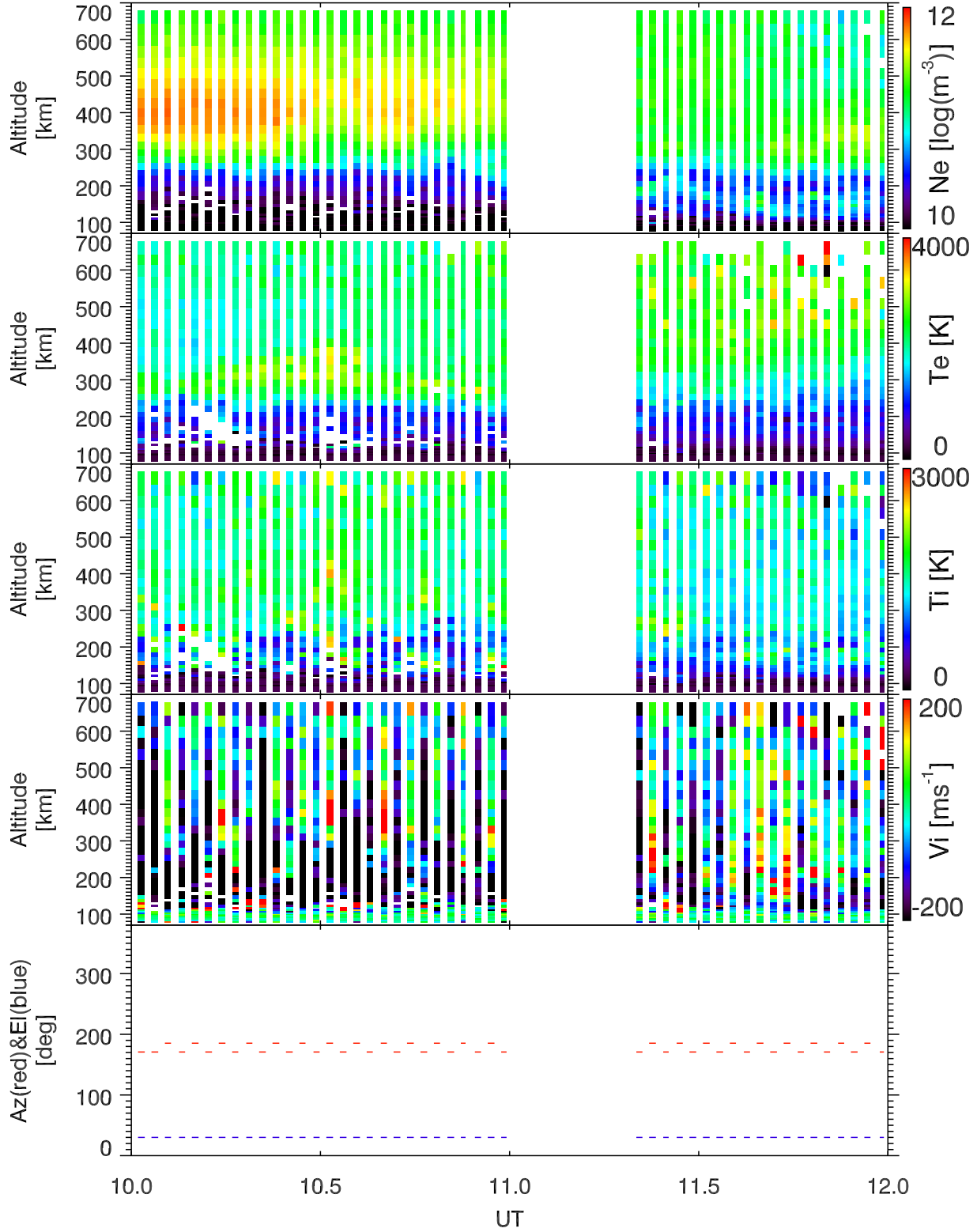
EISCAT 2001-12-12_10_12UT_tau0_ant@32m.
