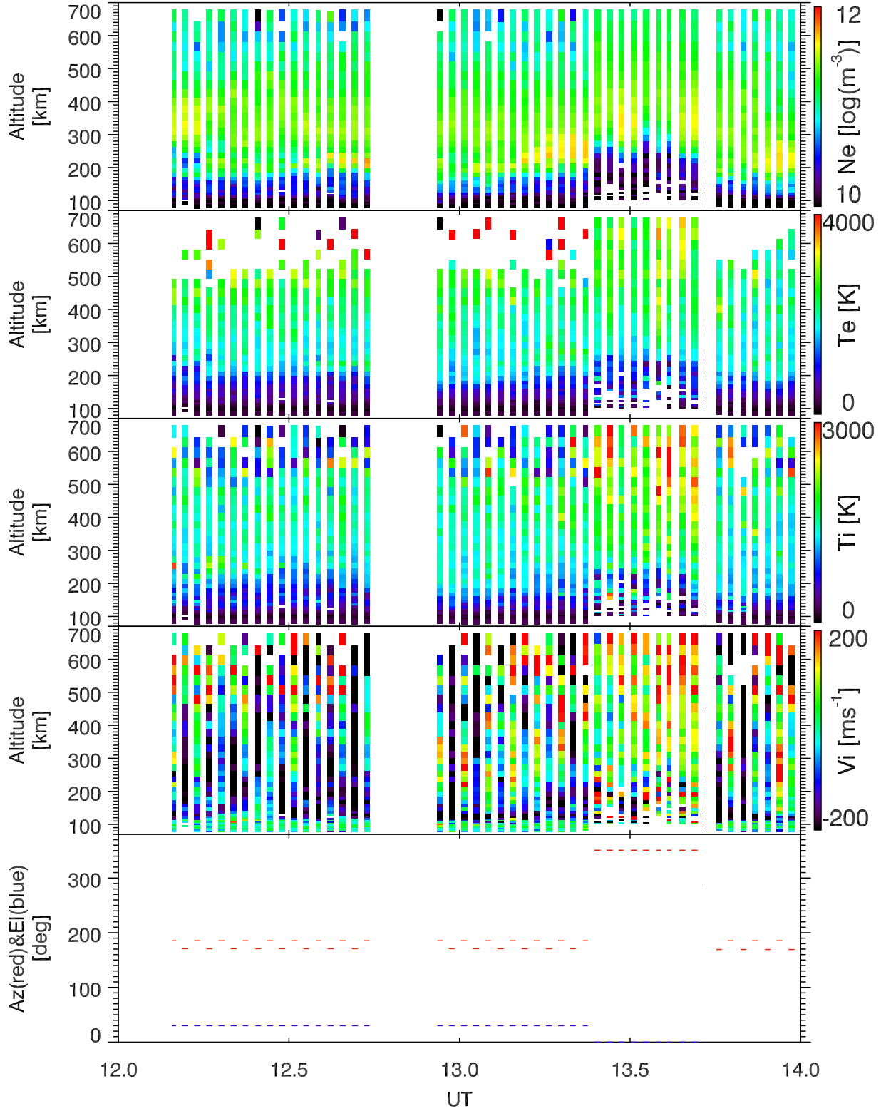
EISCAT 2001-12-12_12_14UT_tau0_ant@32m.
