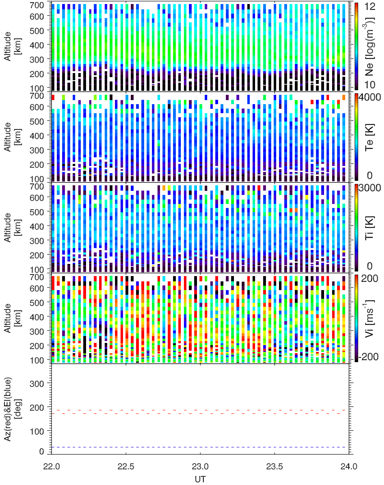
EISCAT 2001-12-13_22_24UT_tau0_ant@32m.
