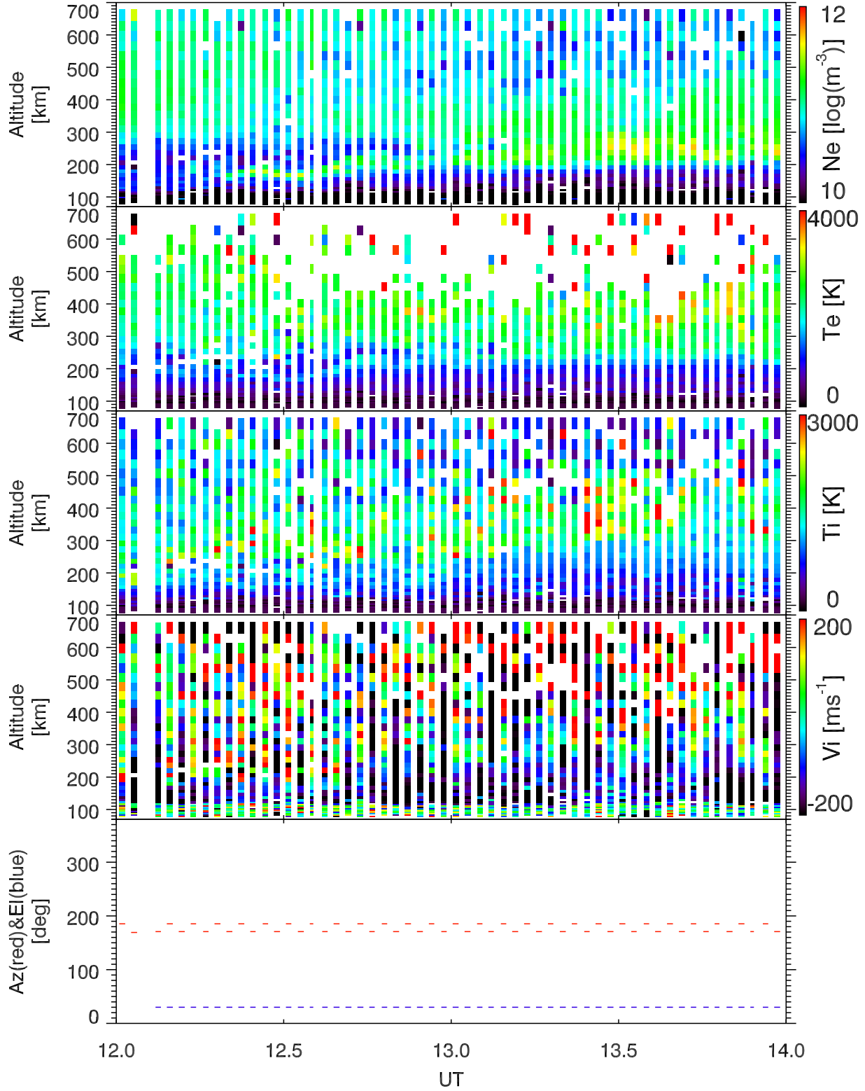
EISCAT 2001-12-14_12_14UT_tau0_ant@32m.
