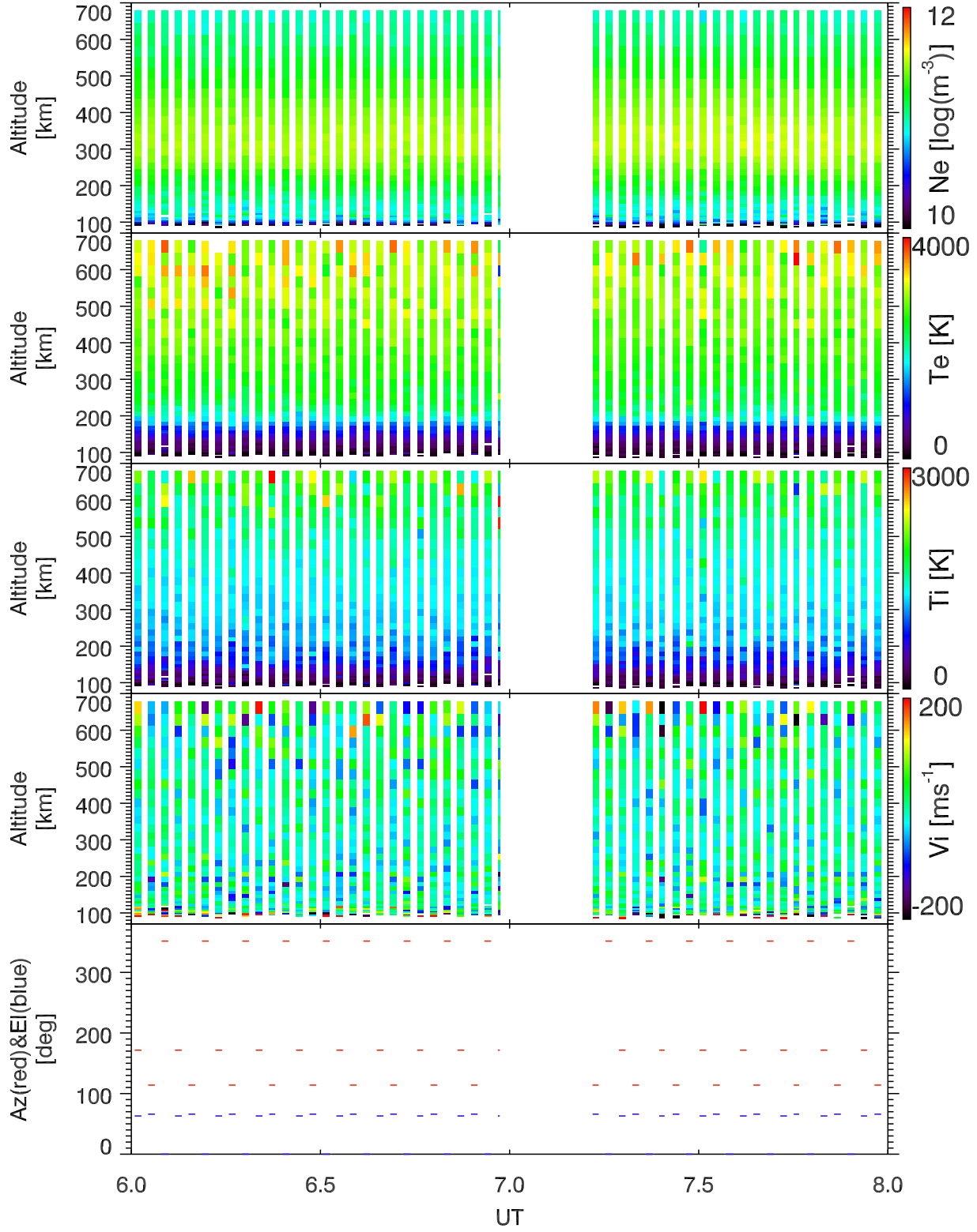
EISCAT 2002-07-31_06_08UT_tau0_ant@32m.
