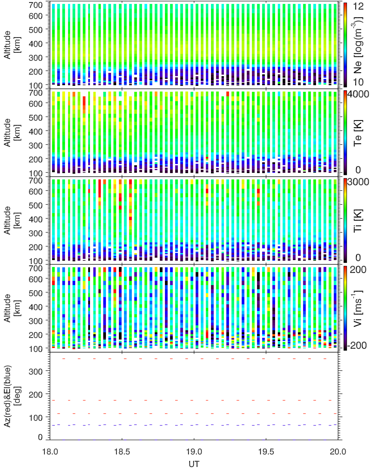
EISCAT 2002-09-13_18_20UT_tau0_ant@32m.
