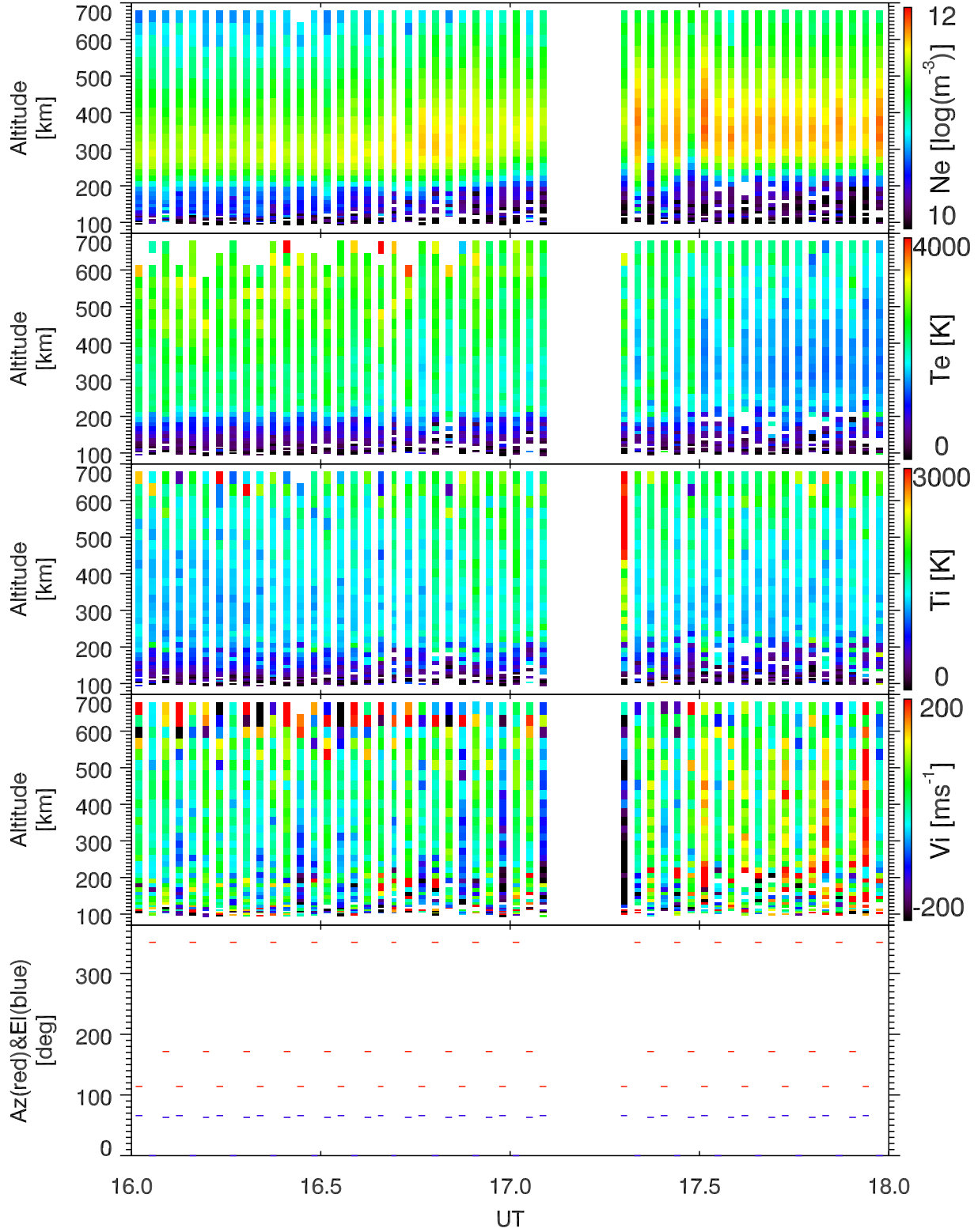
EISCAT 2002-09-26_16_18UT_tau0_ant@32m.
