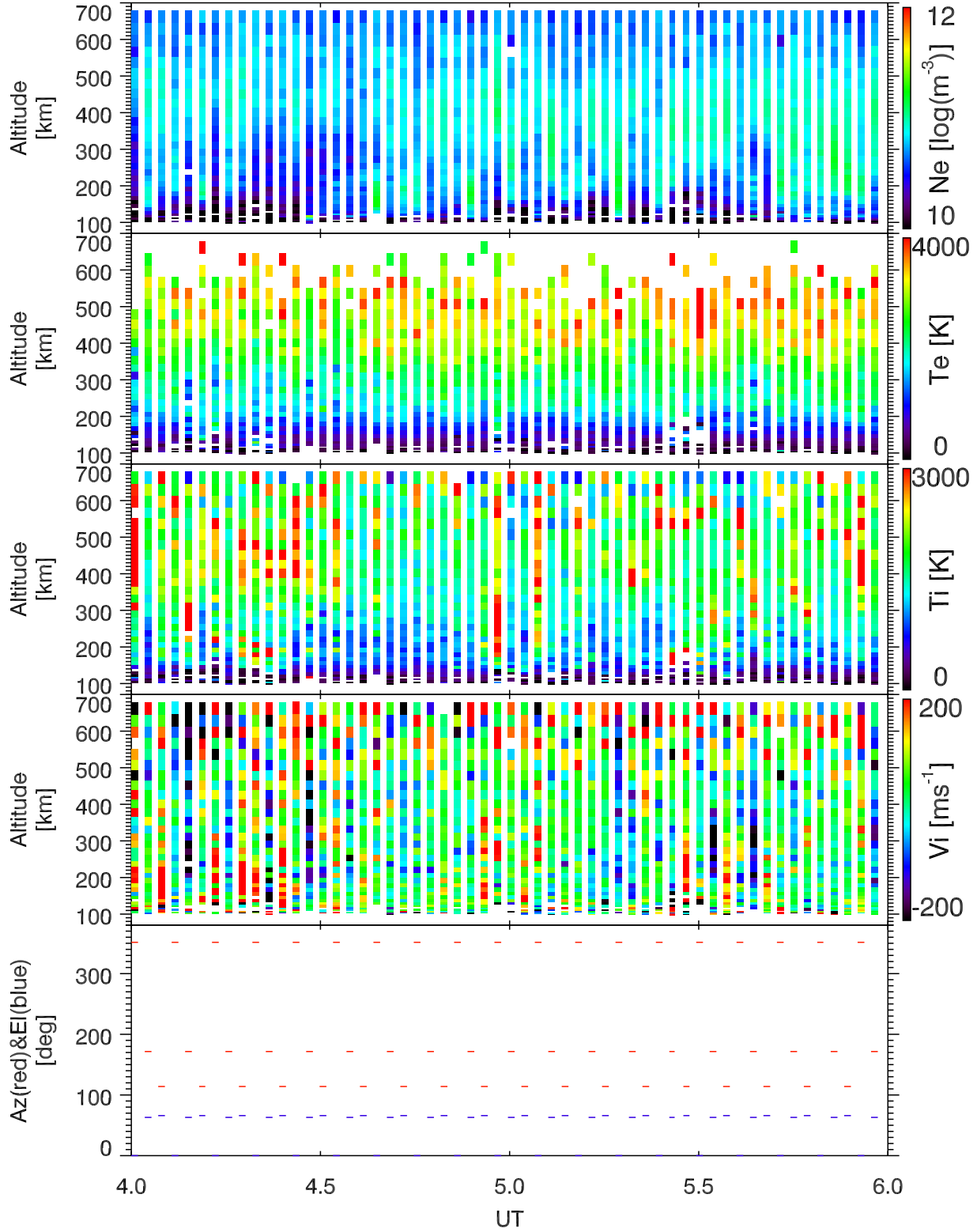
EISCAT 2002-10-12_04_06UT_tau0_ant@32m.
