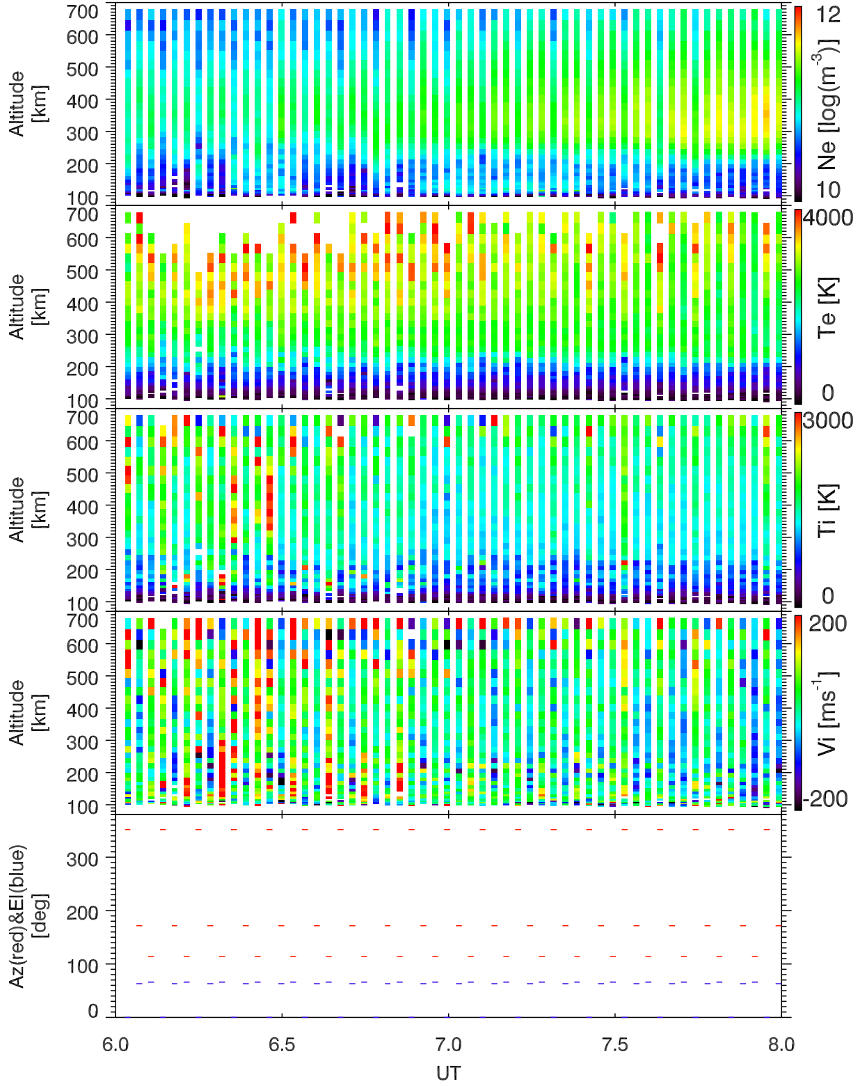
EISCAT 2002-10-12_06_08UT_tau0_ant@32m.
