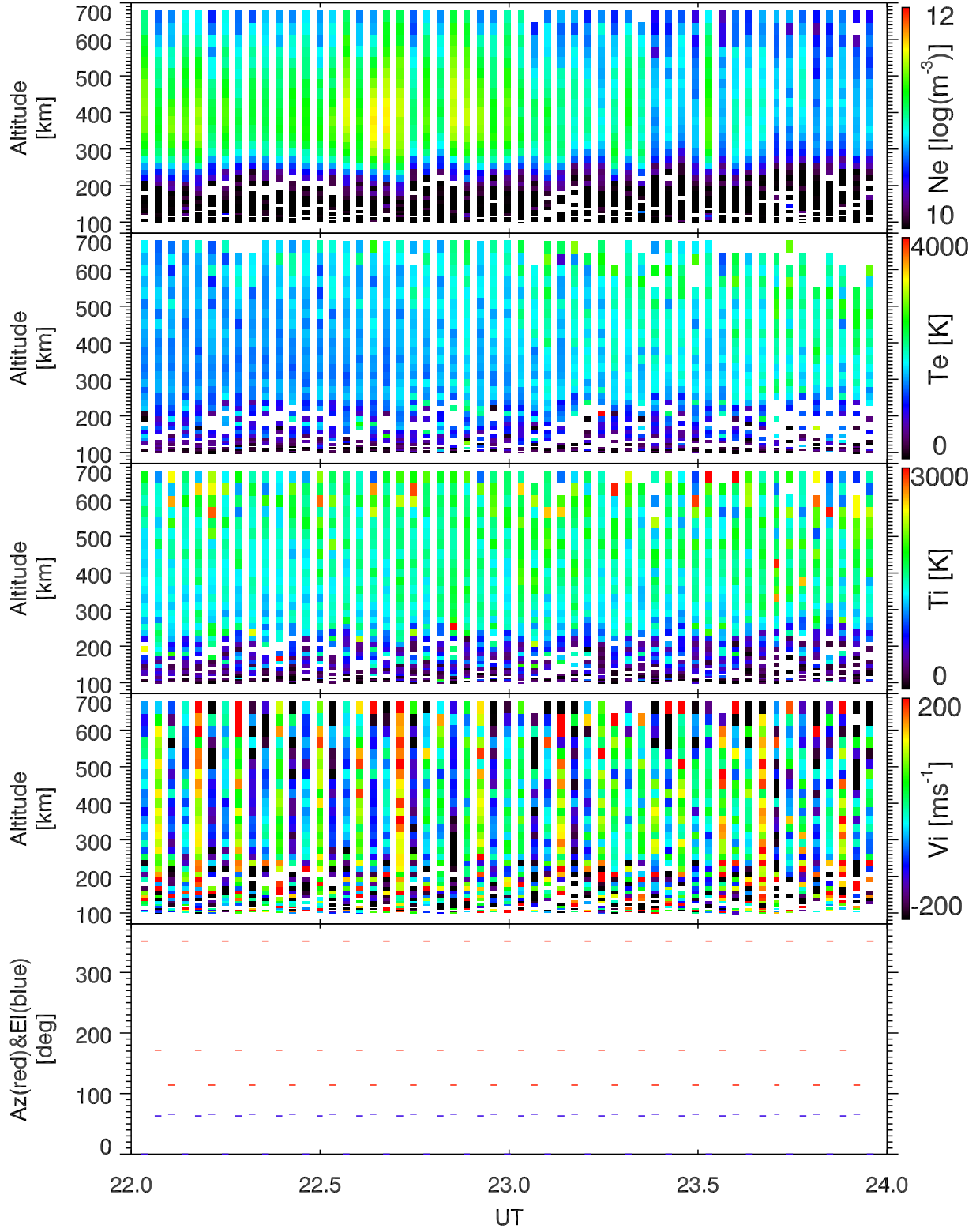
EISCAT 2002-10-12_22_24UT_tau0_ant@32m.
