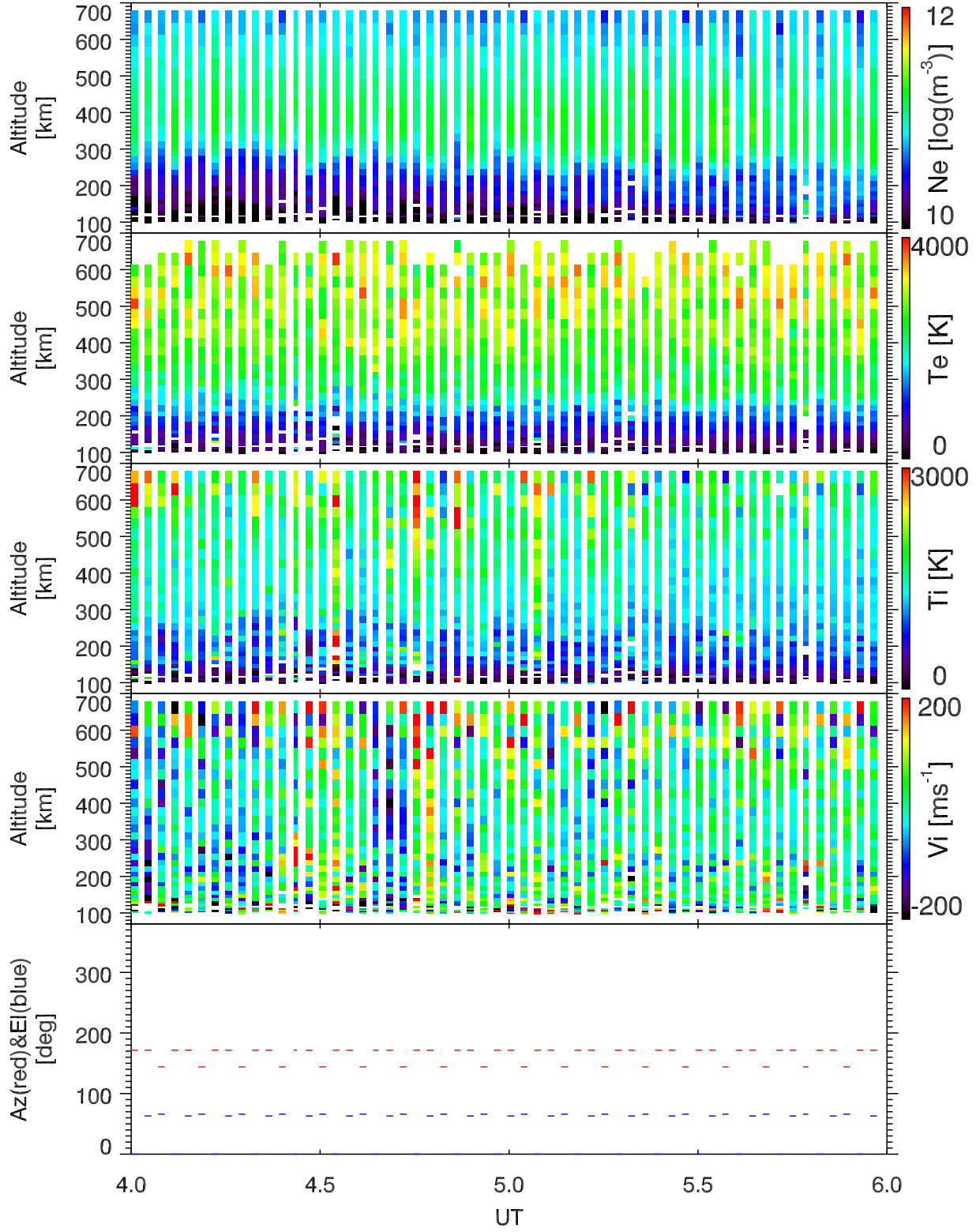
EISCAT 2002-10-16_04_06UT_tau0_ant@32m.
