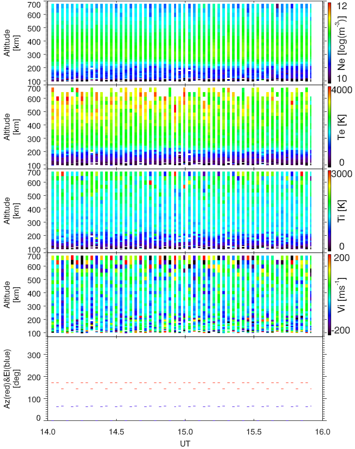
EISCAT 2002-10-16_14_16UT_tau0_ant@32m.
