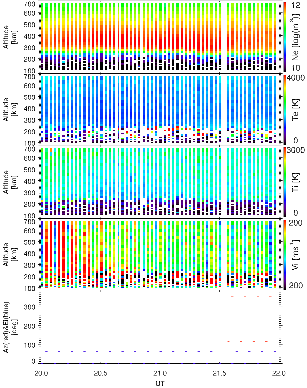
EISCAT 2002-10-16_20_22UT_tau0_ant@32m.
