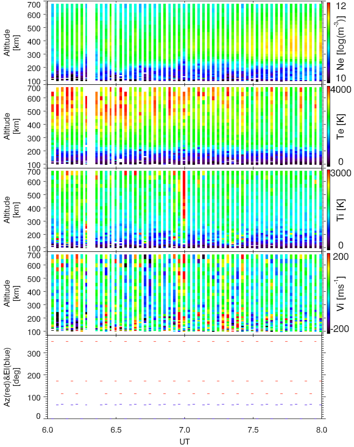
EISCAT 2002-10-17_06_08UT_tau0_ant@32m.
