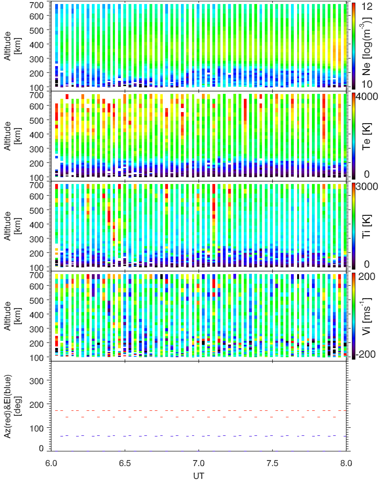
EISCAT 2002-10-19_06_08UT_tau0_ant@32m.
