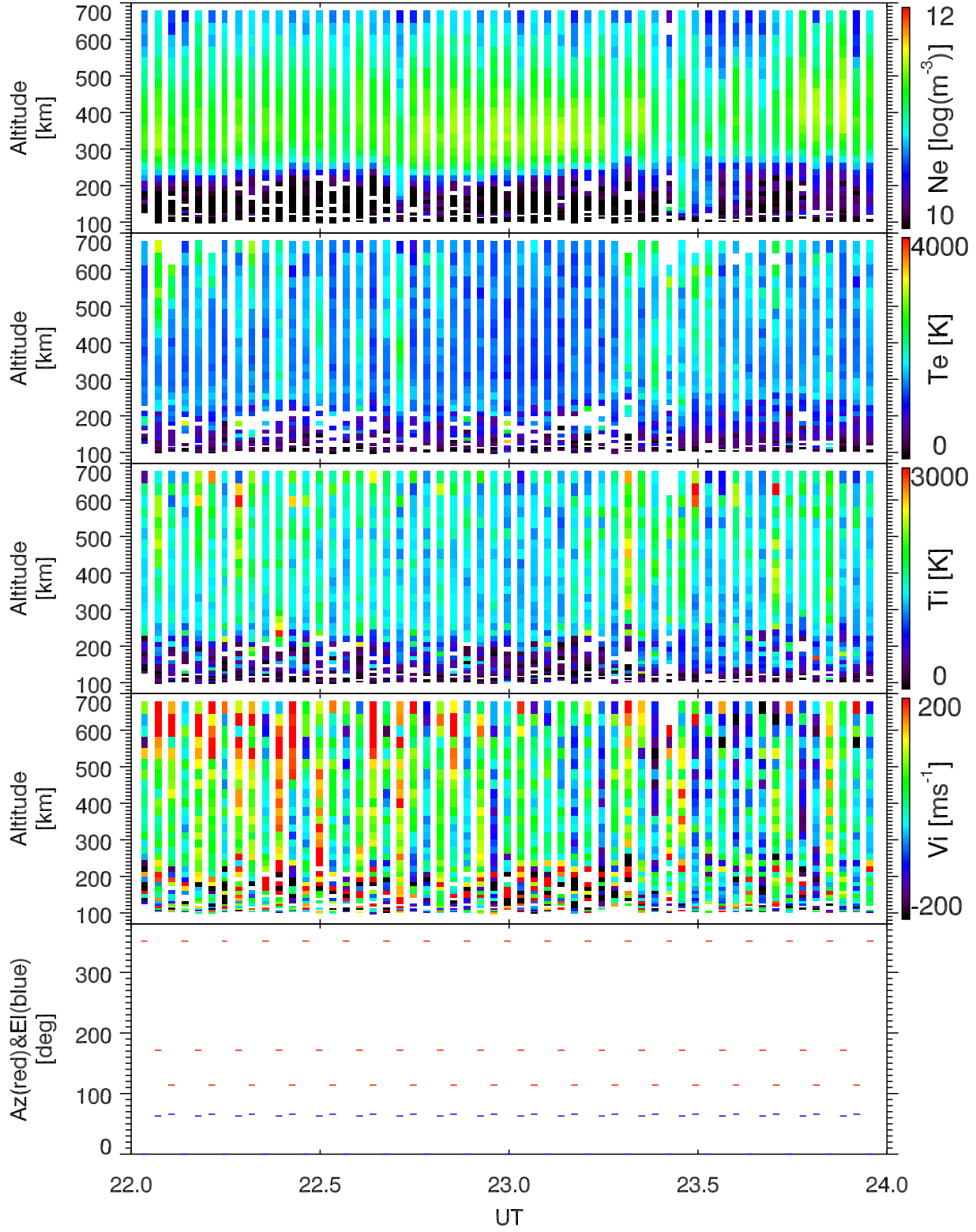
EISCAT 2002-10-20_22_24UT_tau0_ant@32m.
