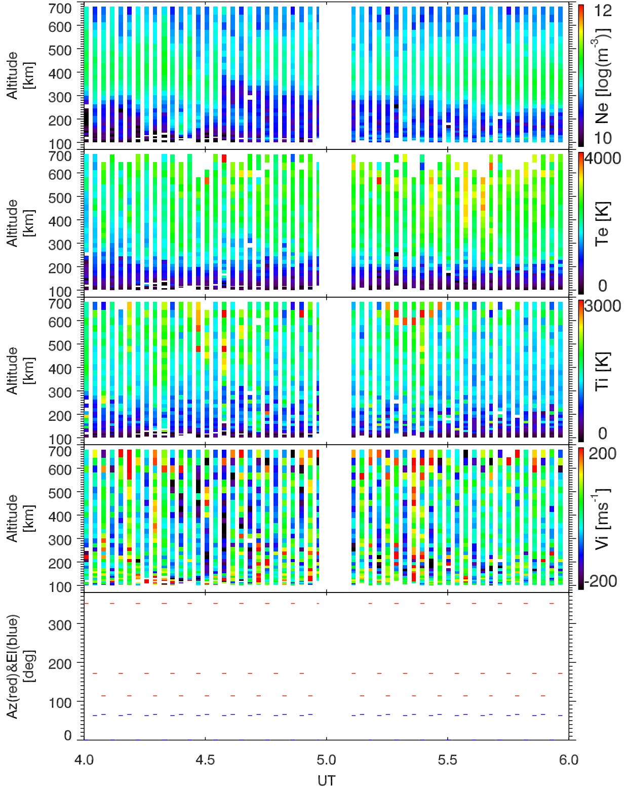
EISCAT 2002-10-21_04_06UT_tau0_ant@32m.
