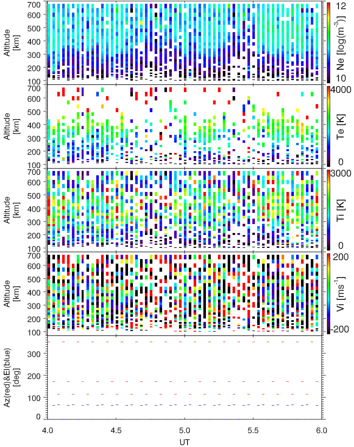
EISCAT 2002-10-25_04_06UT_tau0_ant@32m.
