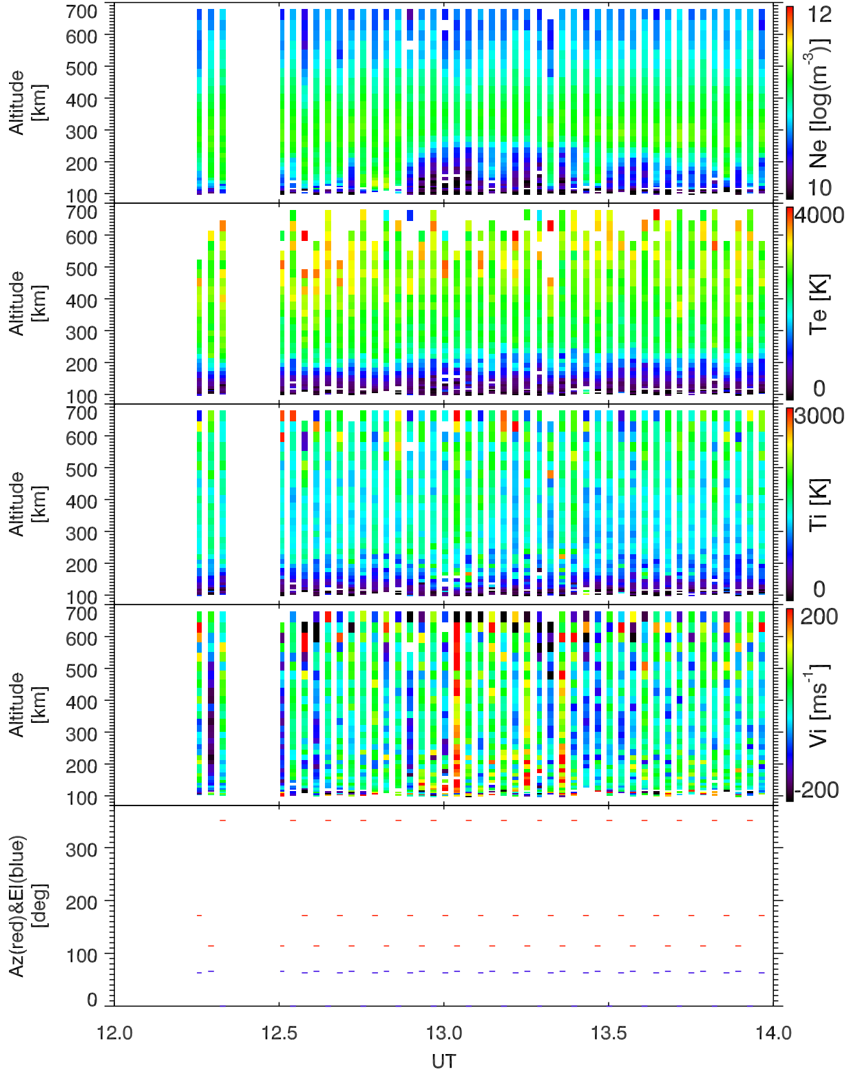
EISCAT 2002-10-28_12_14UT_tau0_ant@32m.
