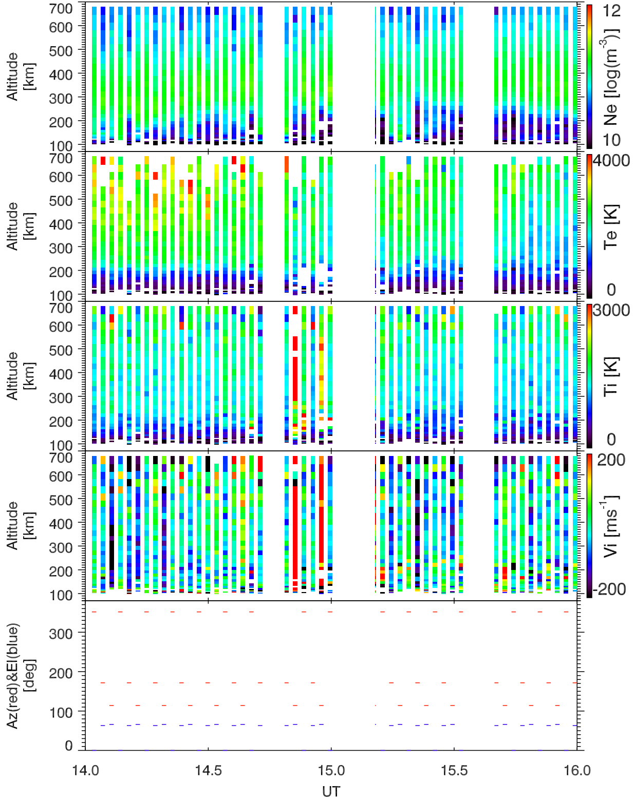
EISCAT 2002-10-28_14_16UT_tau0_ant@32m.
