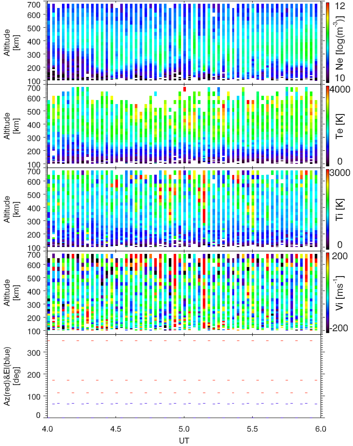
EISCAT 2002-11-01_04_06UT_tau0_ant@32m.
