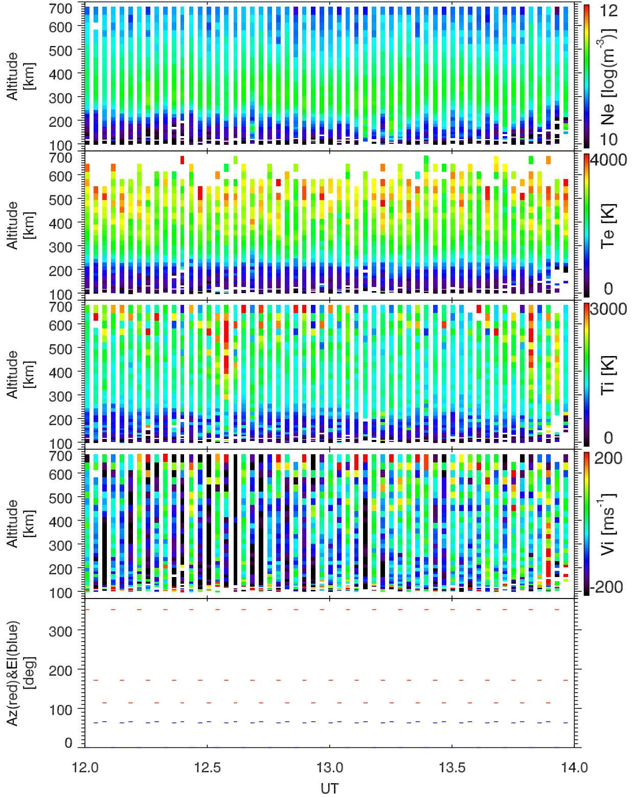
EISCAT 2002-11-02_12_14UT_tau0_ant@32m.
