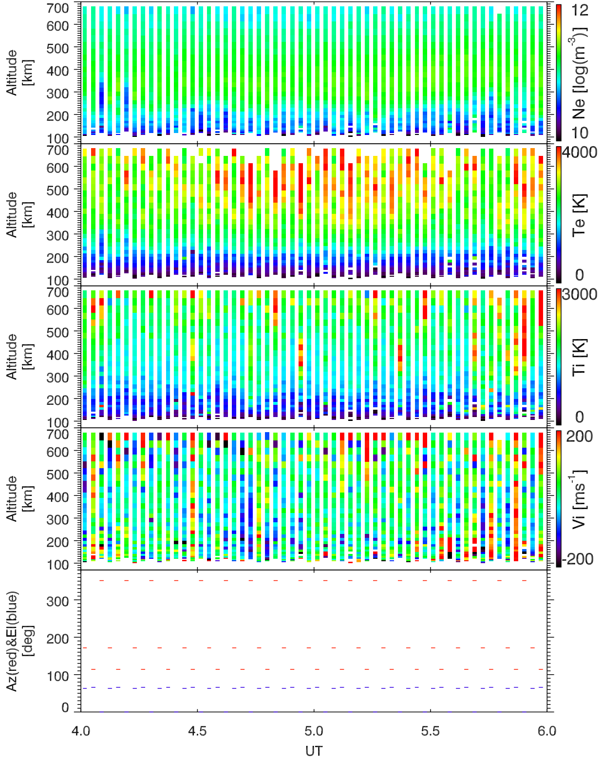
EISCAT 2002-11-12_04_06UT_tau0_ant@32m.
