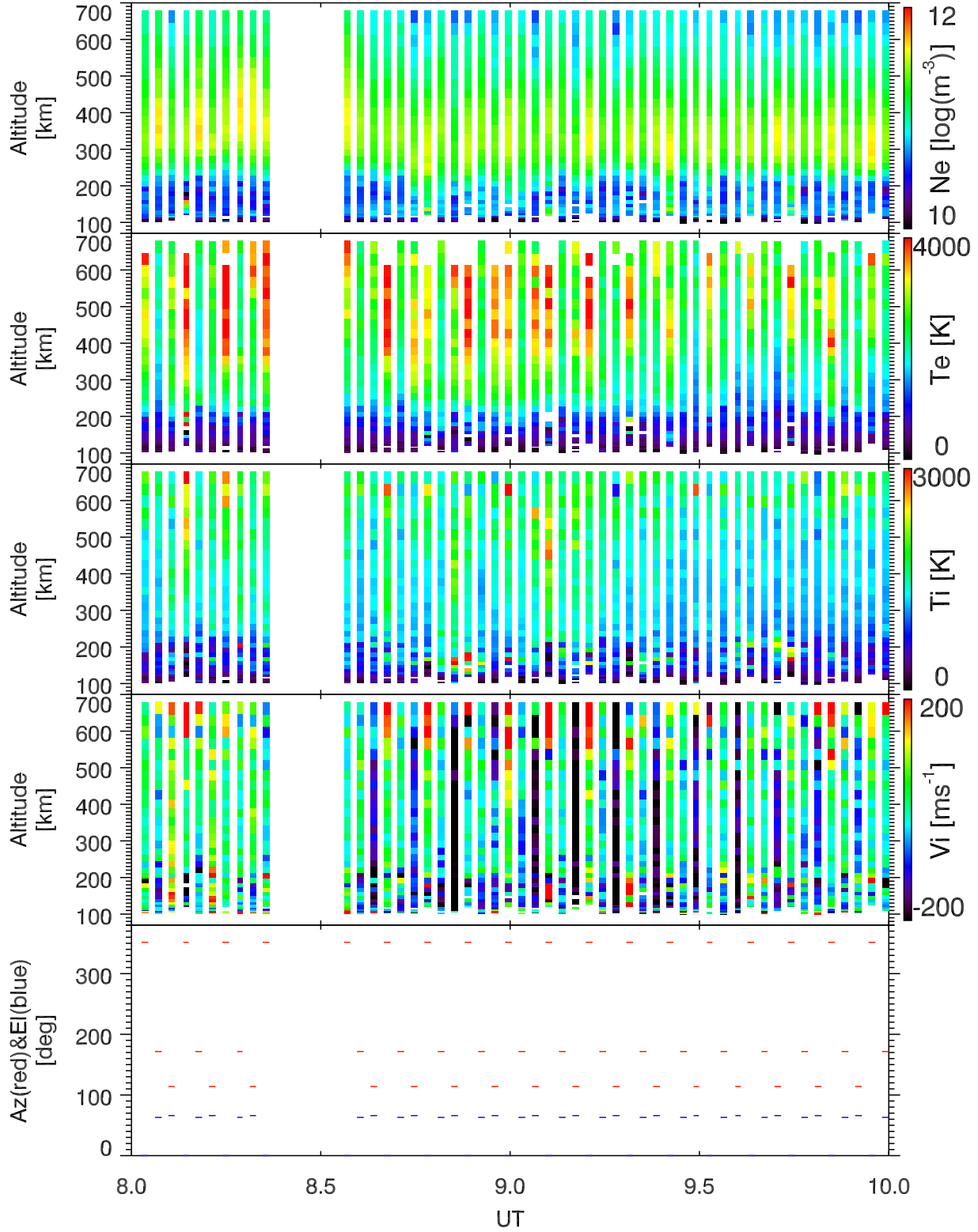
EISCAT 2002-11-12_08_10UT_tau0_ant@32m.
