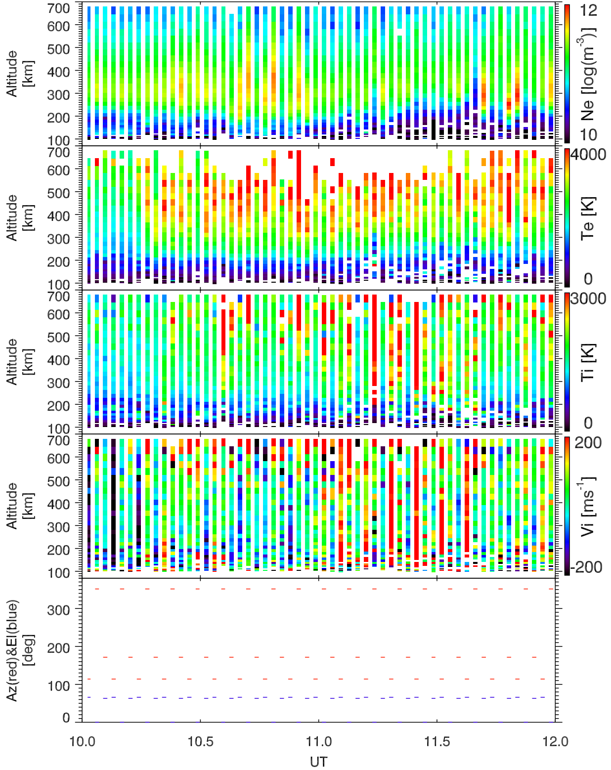
EISCAT 2002-11-12_10_12UT_tau0_ant@32m.
