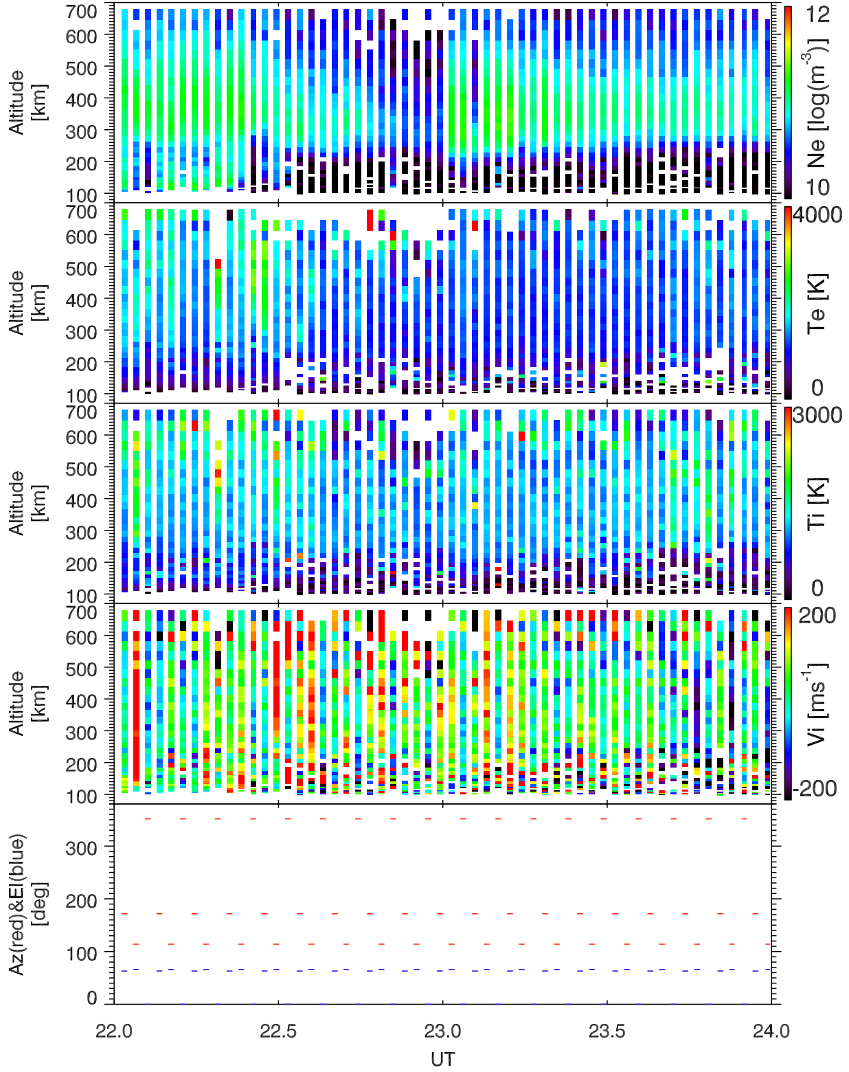
EISCAT 2002-11-13_22_24UT_tau0_ant@32m.
